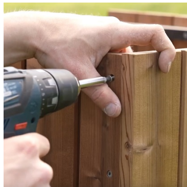
Abbildung 19: Lieferumfang, Verschrauben der Wände, Deckel auflegen
