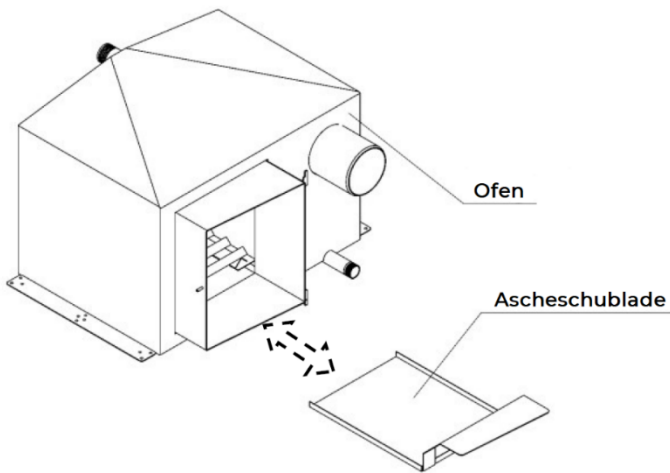
Abbildung 30: Darstellung des Ofens und der Ascheschublade (hier: ohne Edelstahlverkleidung)
