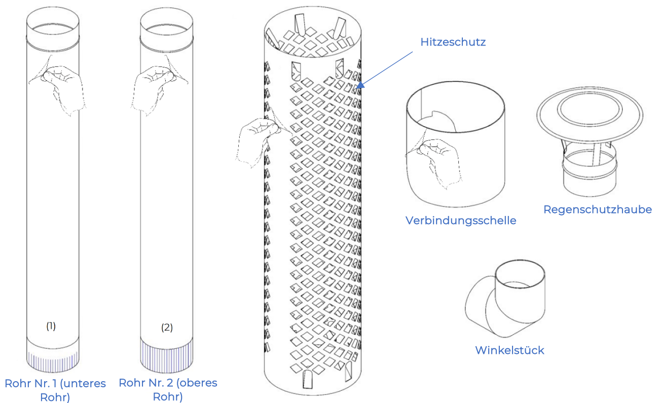
Abbildung 13: Lieferumfang des Abzugsrohres
