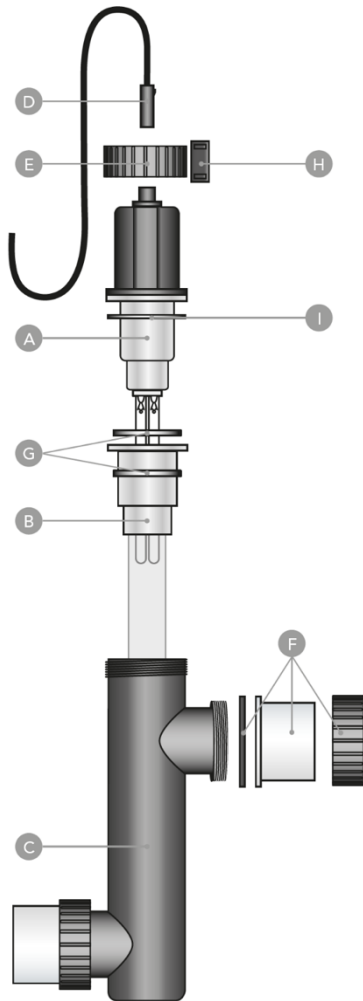
Abbildung 29: Details der UV-Lampe
