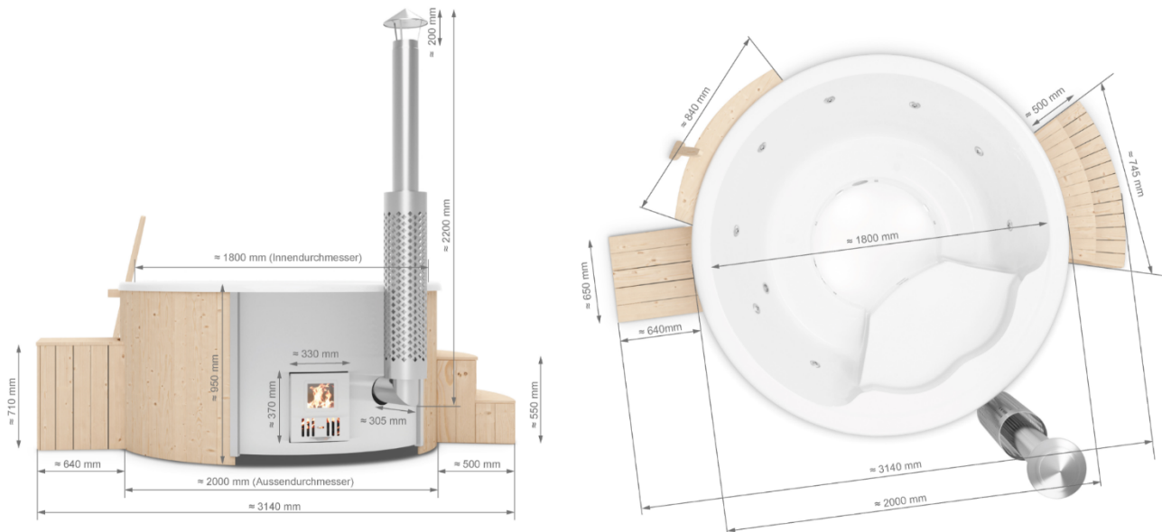
Abbildung 8: Maße des Hot Tubs 180, Ausführungsvariante „SAPHIR“
